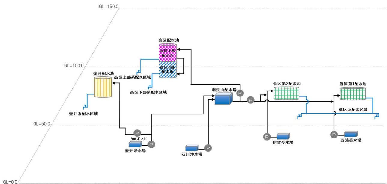
図 2 送配水系統図
