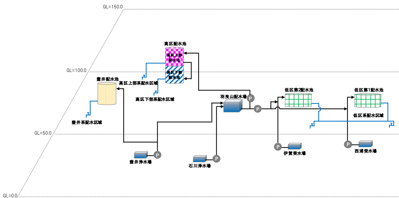
図2 送配水系統図
