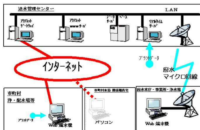
アクアネット大阪のシステム概要図
